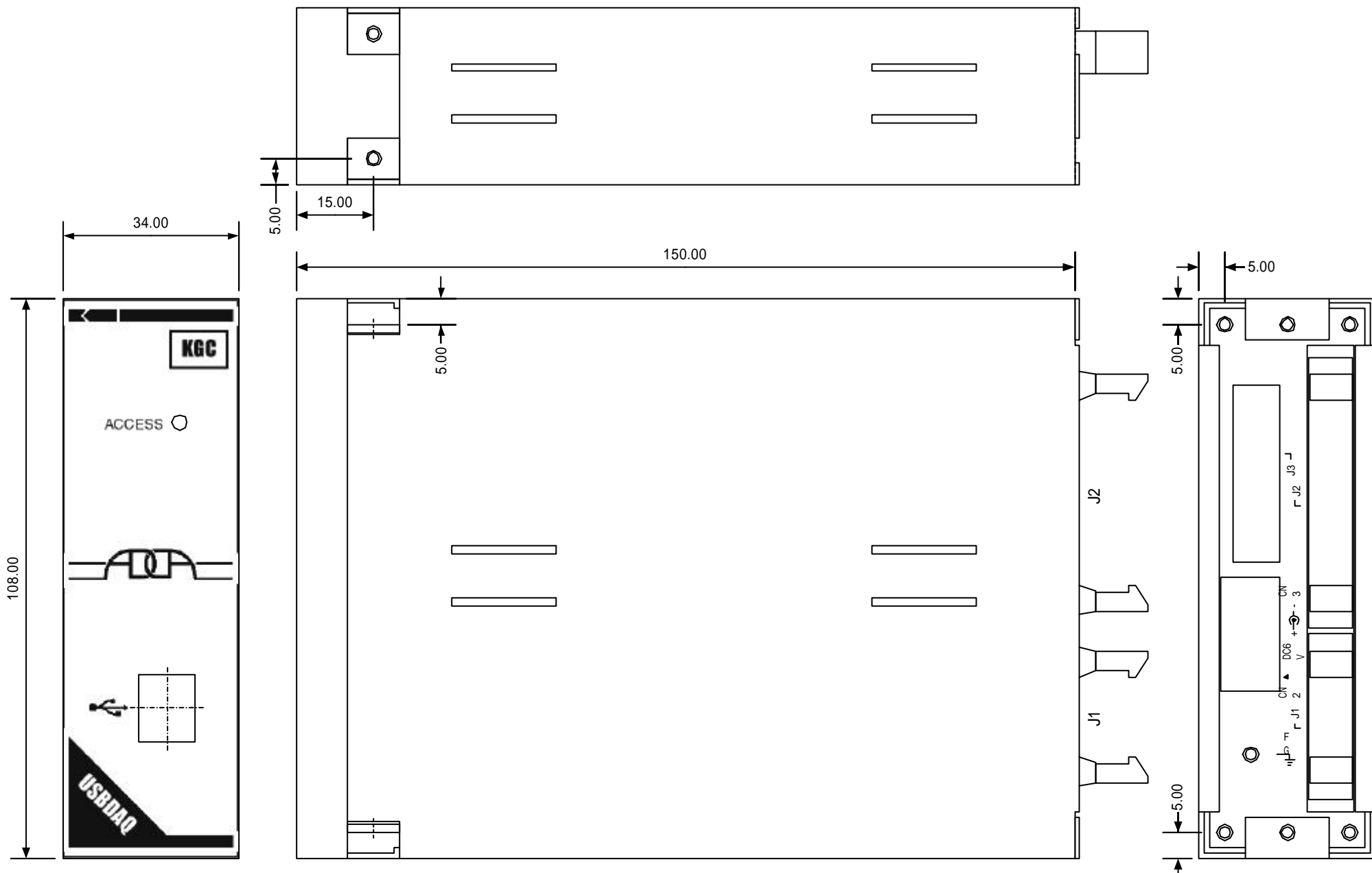
タイトル HKS-0200外形図
